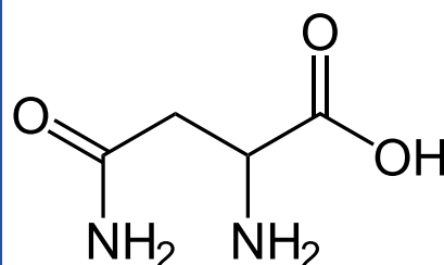
Asparagine
