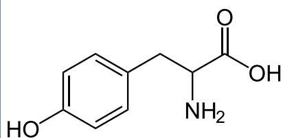
Tyrosine
